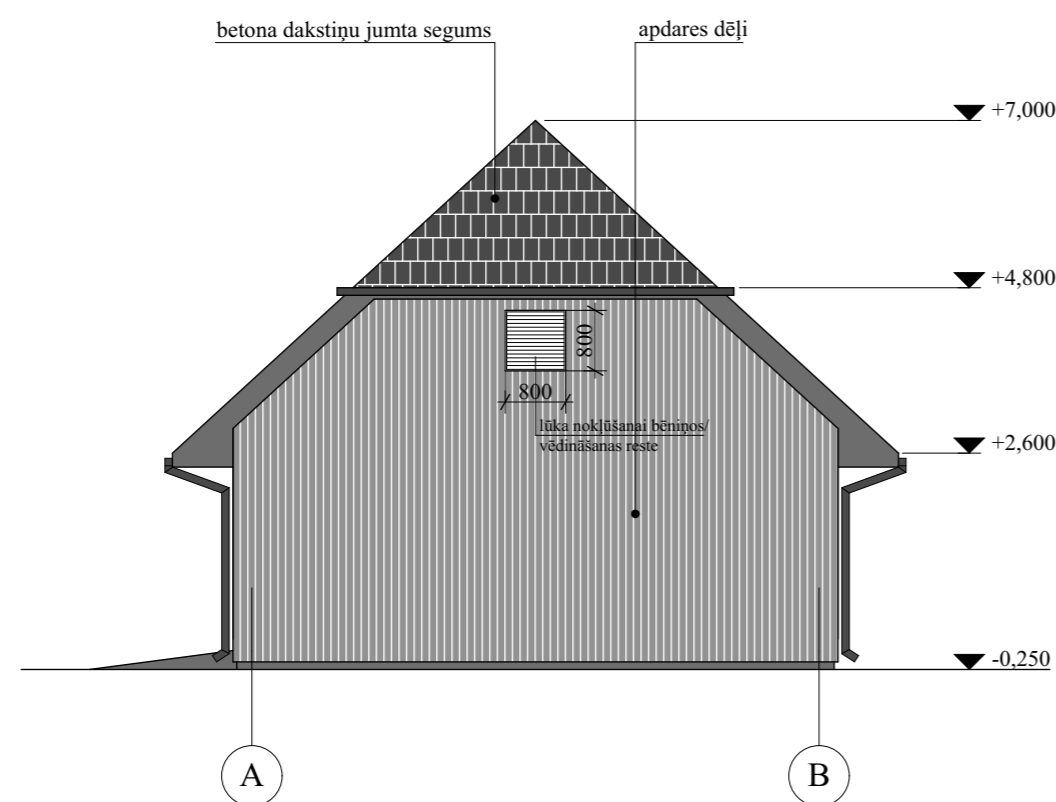
Fasāde asīs A-B
