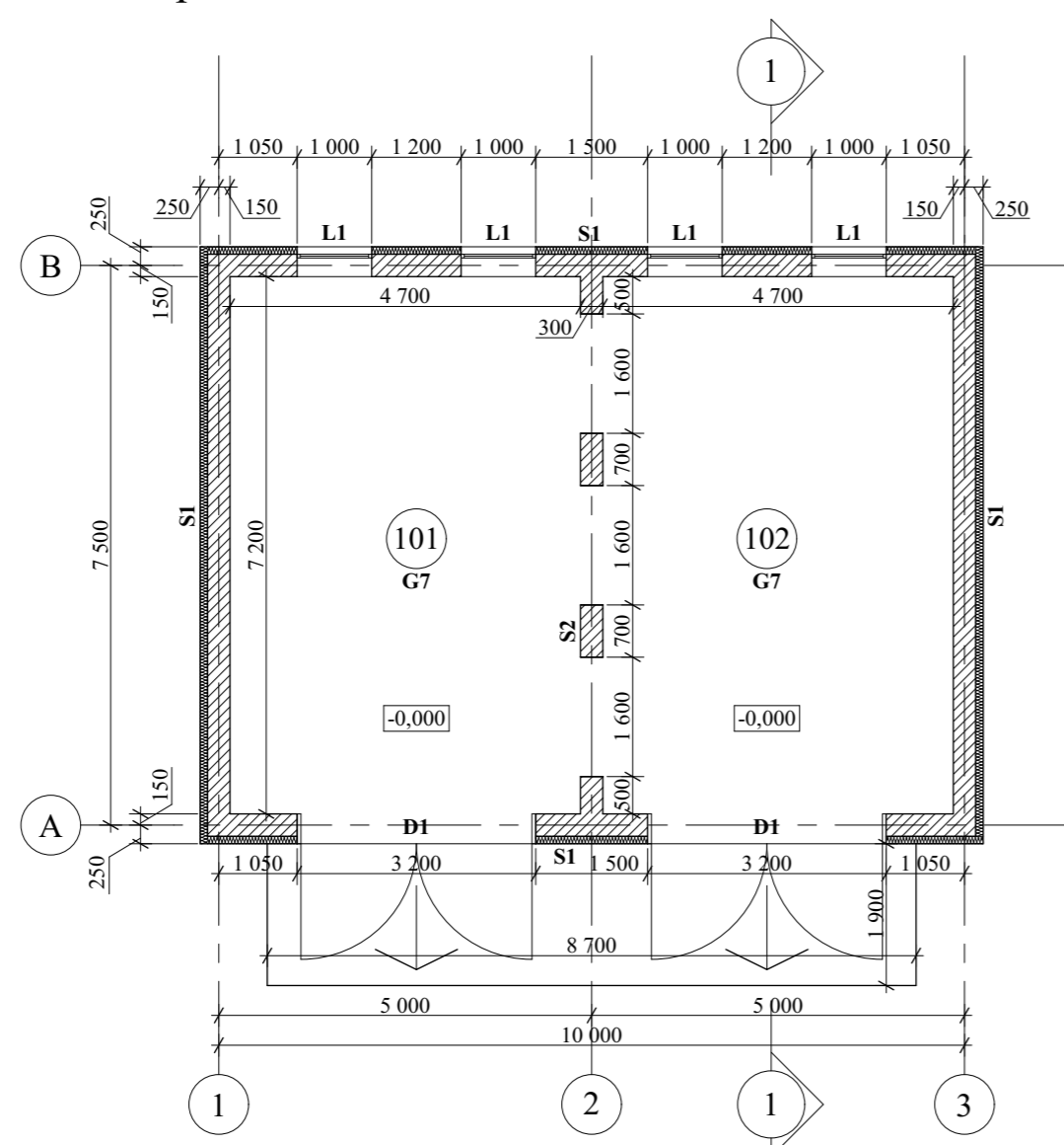
Garāžas plāns
