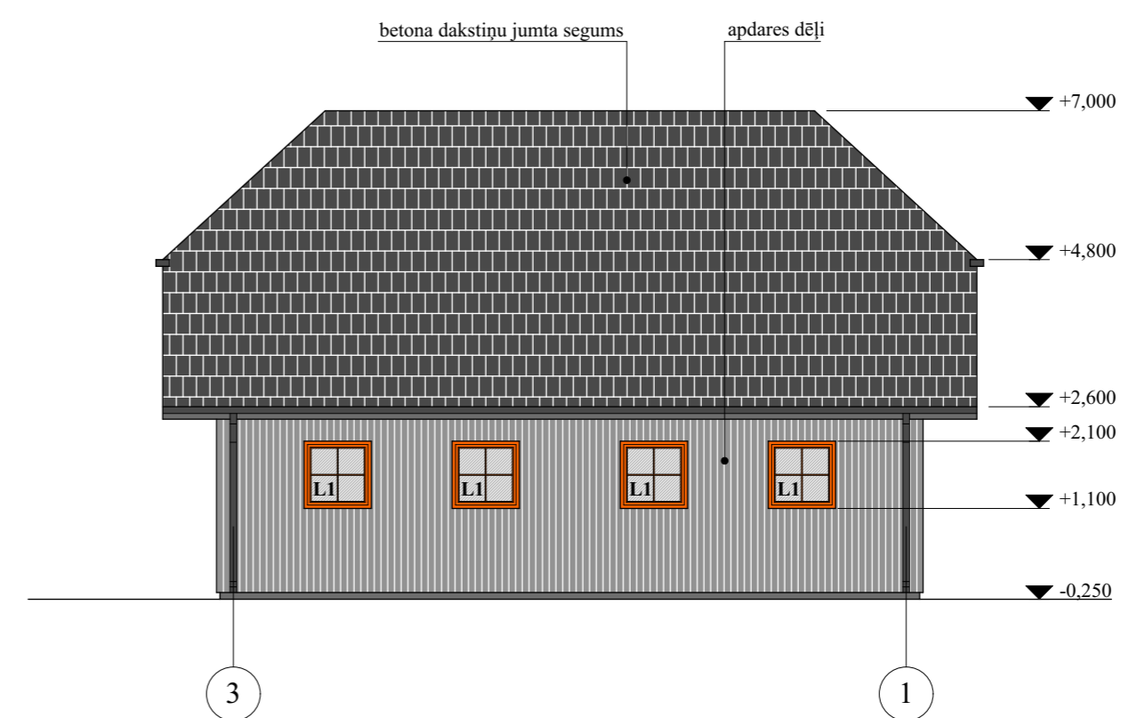
Fasāde asīs 3-1
