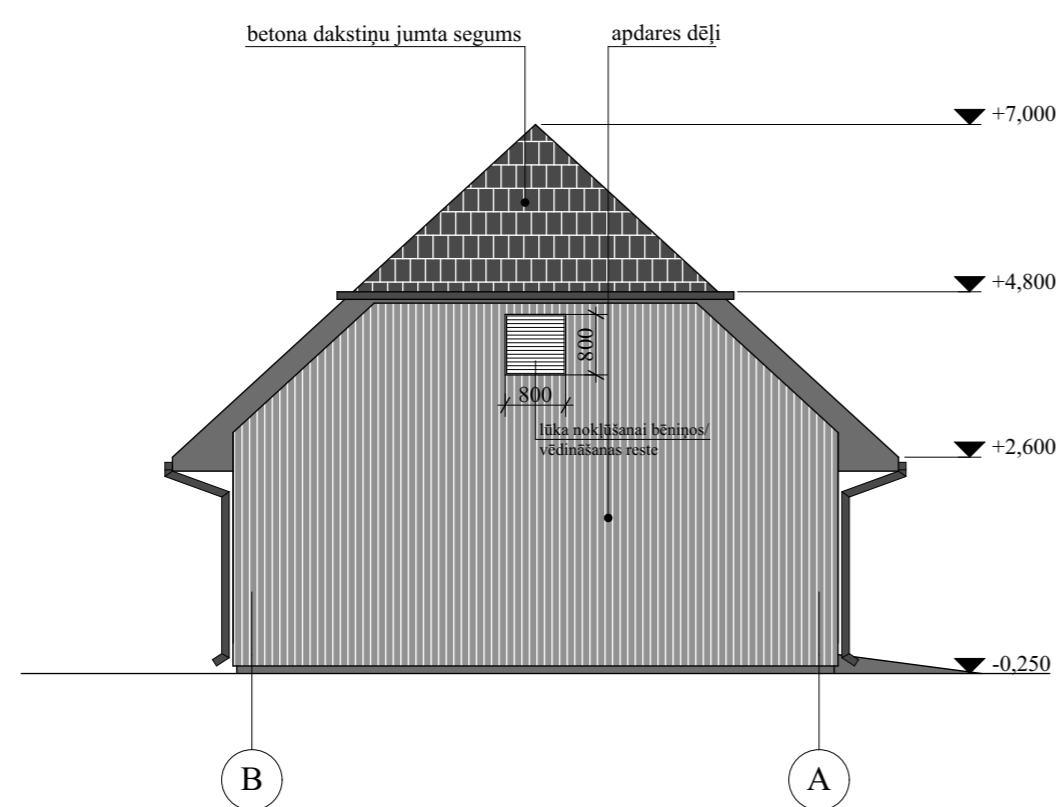
Fasāde asīs B-A
